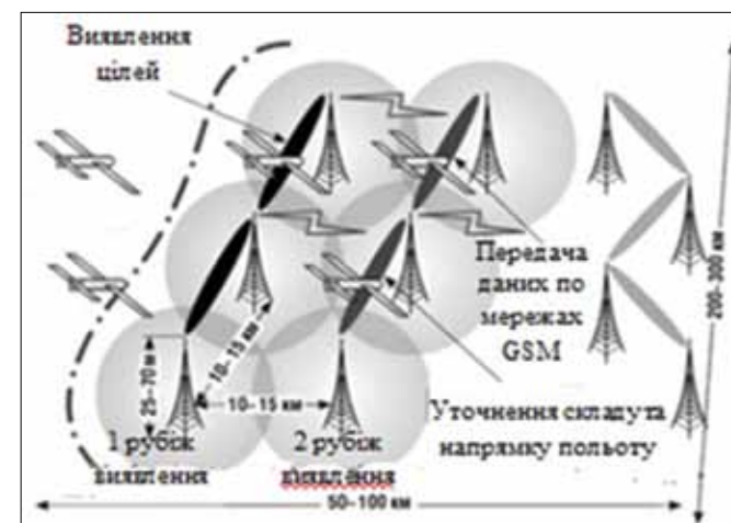
Рис. 2 – Багатопозиційна рознесена радіолокаційна система в полі випромінювання системи осередкового зв'язку
