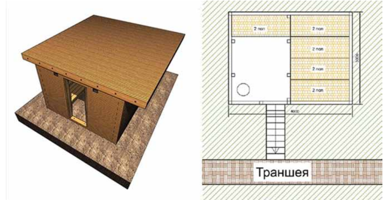
Фото 13. Типове укриття проекту «Народний бліндаж». (Малюнок з сайту http://www.peoplesproject.com/blindage/ )
